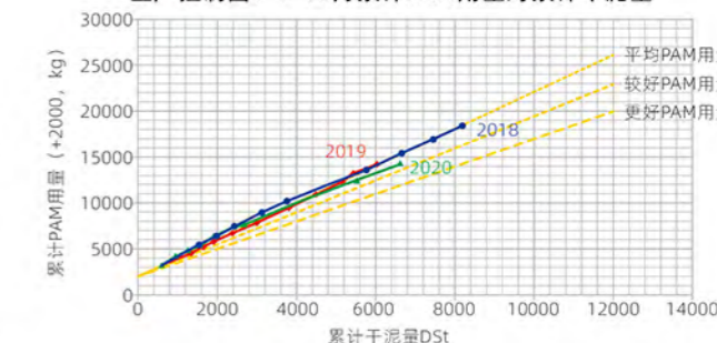
生产控制图：1-10月累计PAM用量对累计干泥量
